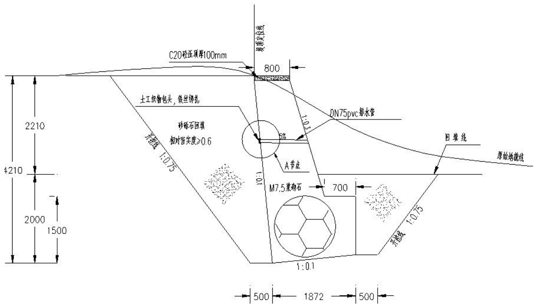
图 1.1 项目河堤断面图
