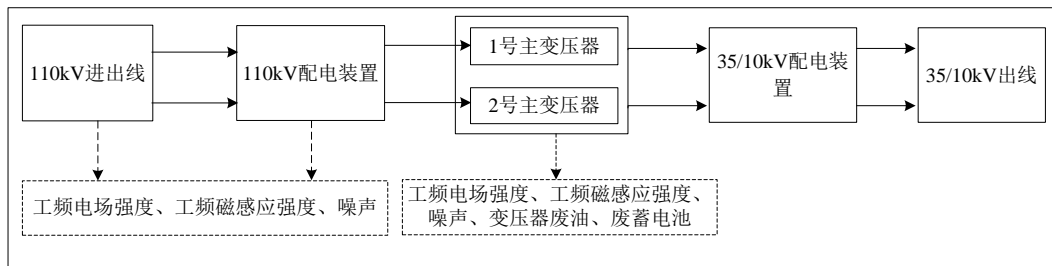
图 4-4 变电站运行期工艺流程及产污环节示意图
