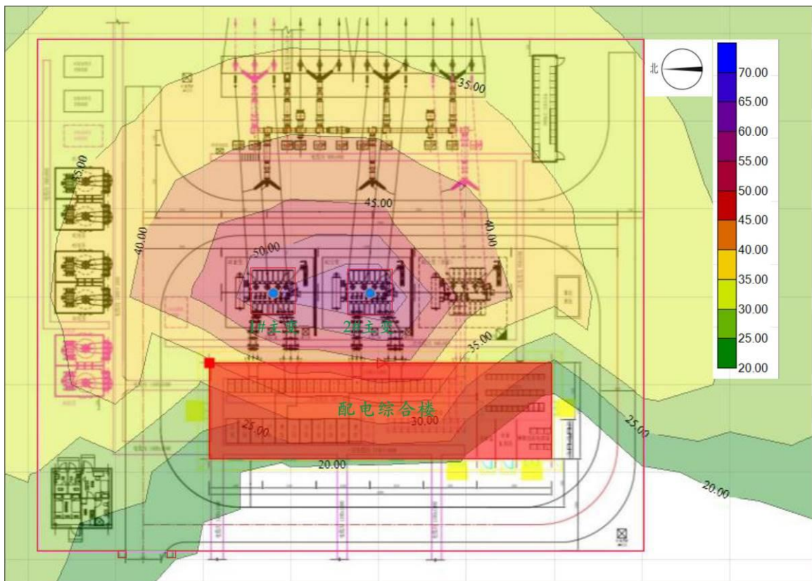
图 4-7 噪声贡献值等值线图
