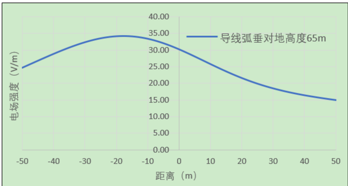
图 6.2-5 单回 JC1 型转角塔电场强度随距离变化趋势
