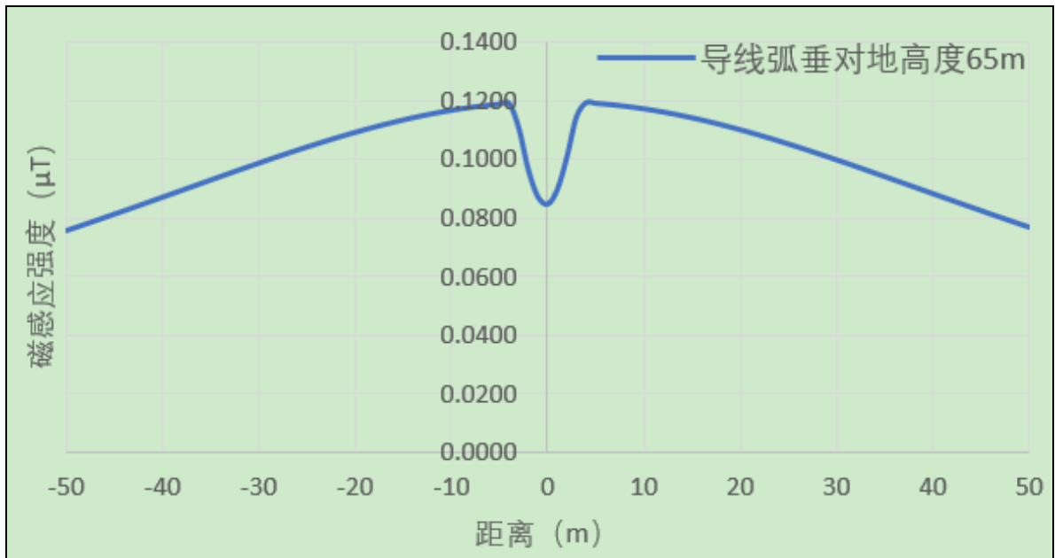
图 6.2-6 单回 JC1 型转角塔磁感应强度随距离变化趋势
