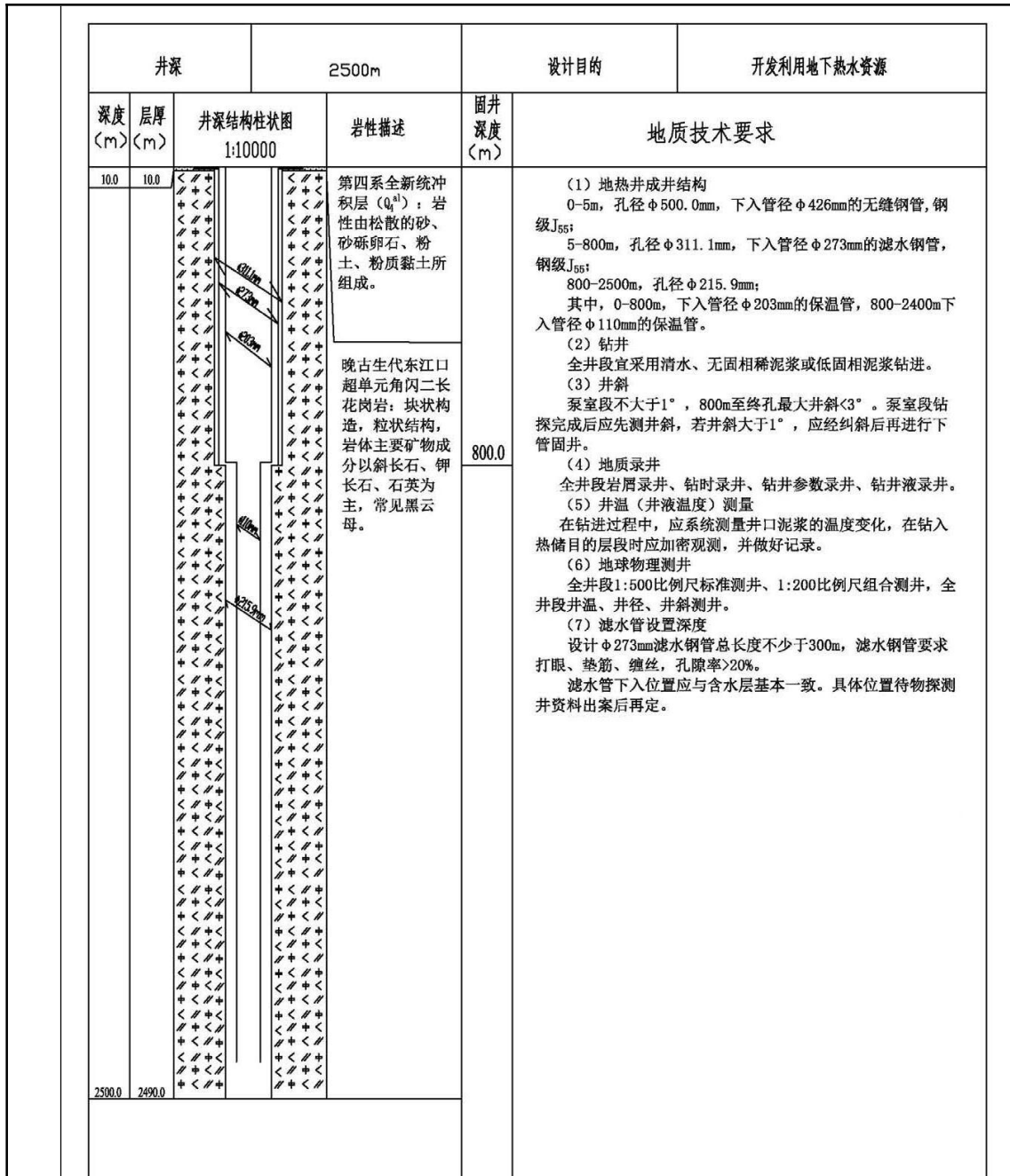
图 2-1 地热井井身结构柱状图
