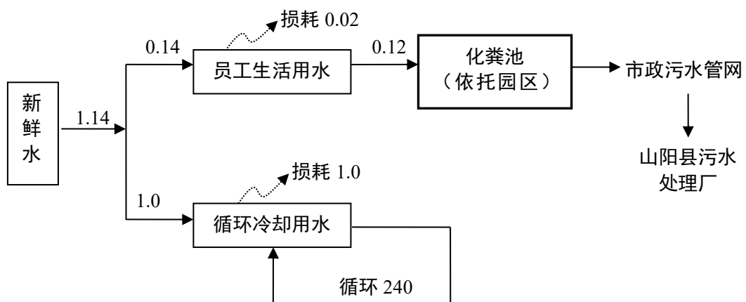
图 2-1 本项目水平衡及污水走向图 (m 3 /d)
