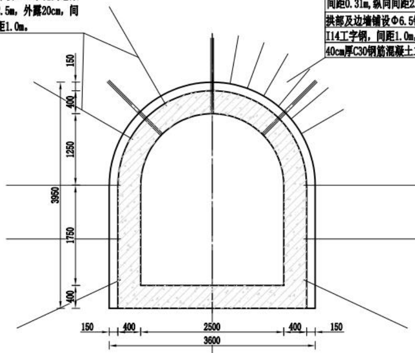
图 2.1-7 IV类围岩隧道结构设计图
