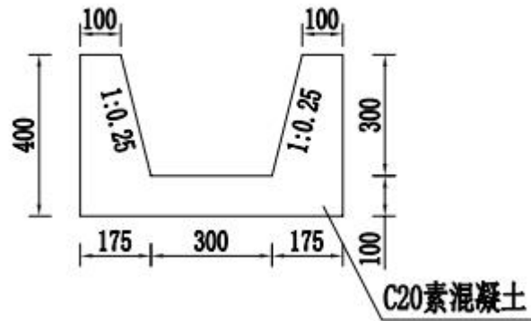
图 2.1-3 隧洞进出口截流沟设计图
