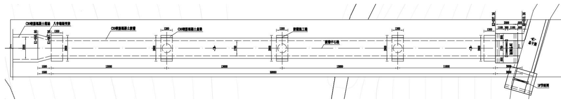
图 2.1-9 波槽平面布置图
