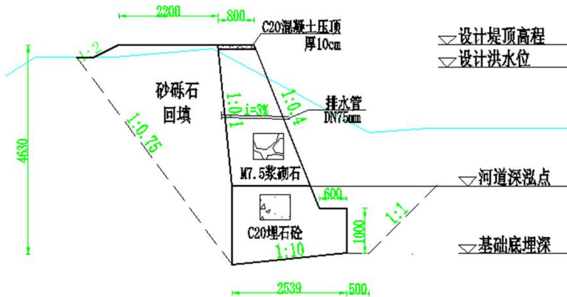
图 2-1 浆砌石仰斜式挡墙结构图
